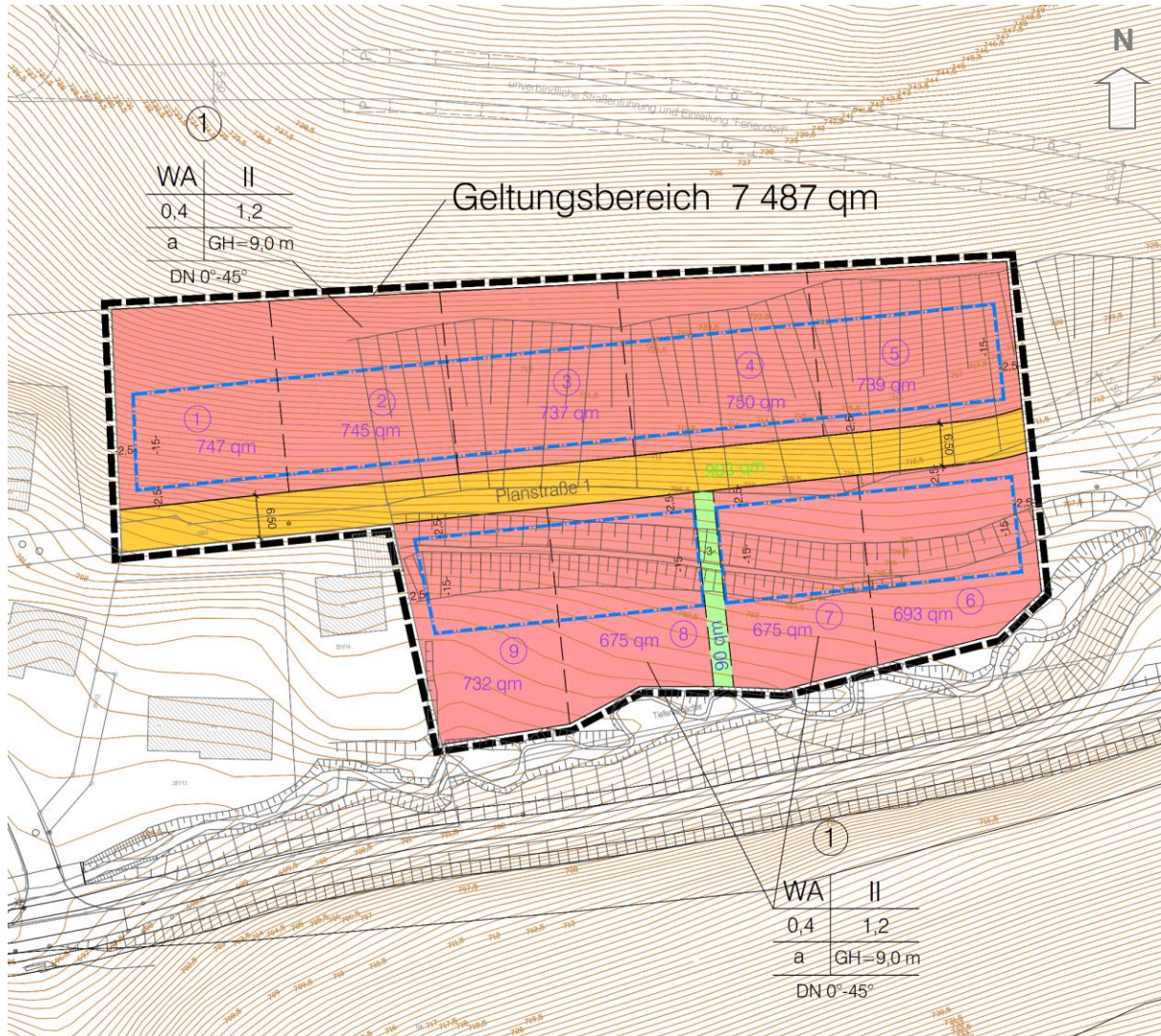
Abbildung 7 - BP „Tiefental“ (Auszug) o. M.
