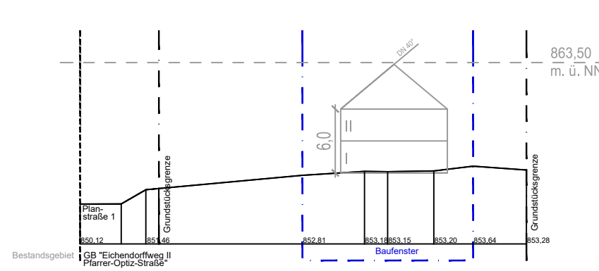
Schnitt B-B
