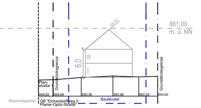
Schnitt D-D
