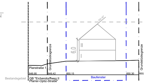
Schnitt C-C
